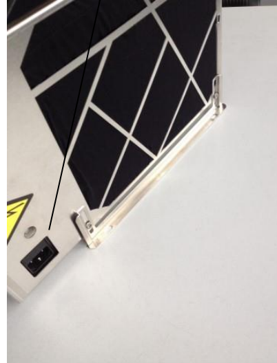
Afb. 9: C14 stroomaansluiting
